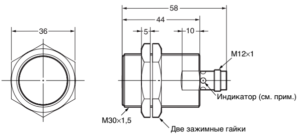
E2A-M30KS15-M1-□□/E2A-S30KS15-M1-□
