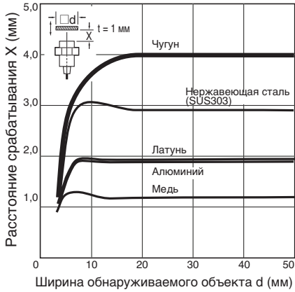
E2A-S08□N04
