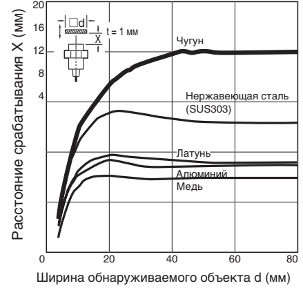
E2A-M18□N16/E2A-S18□N16
